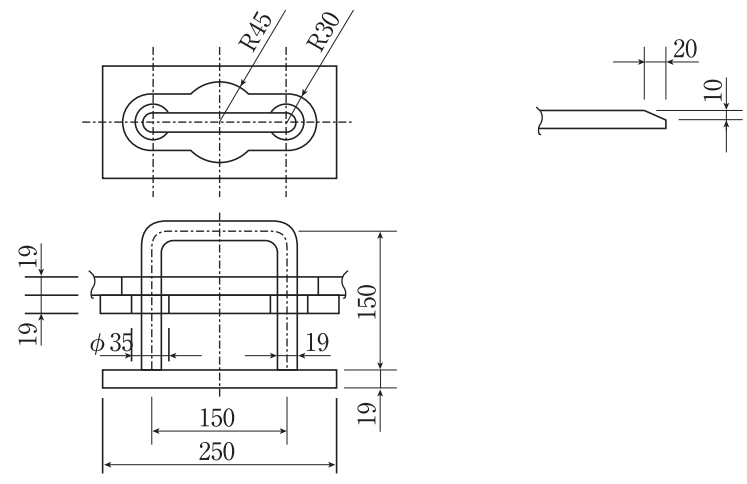
■把手詳細
