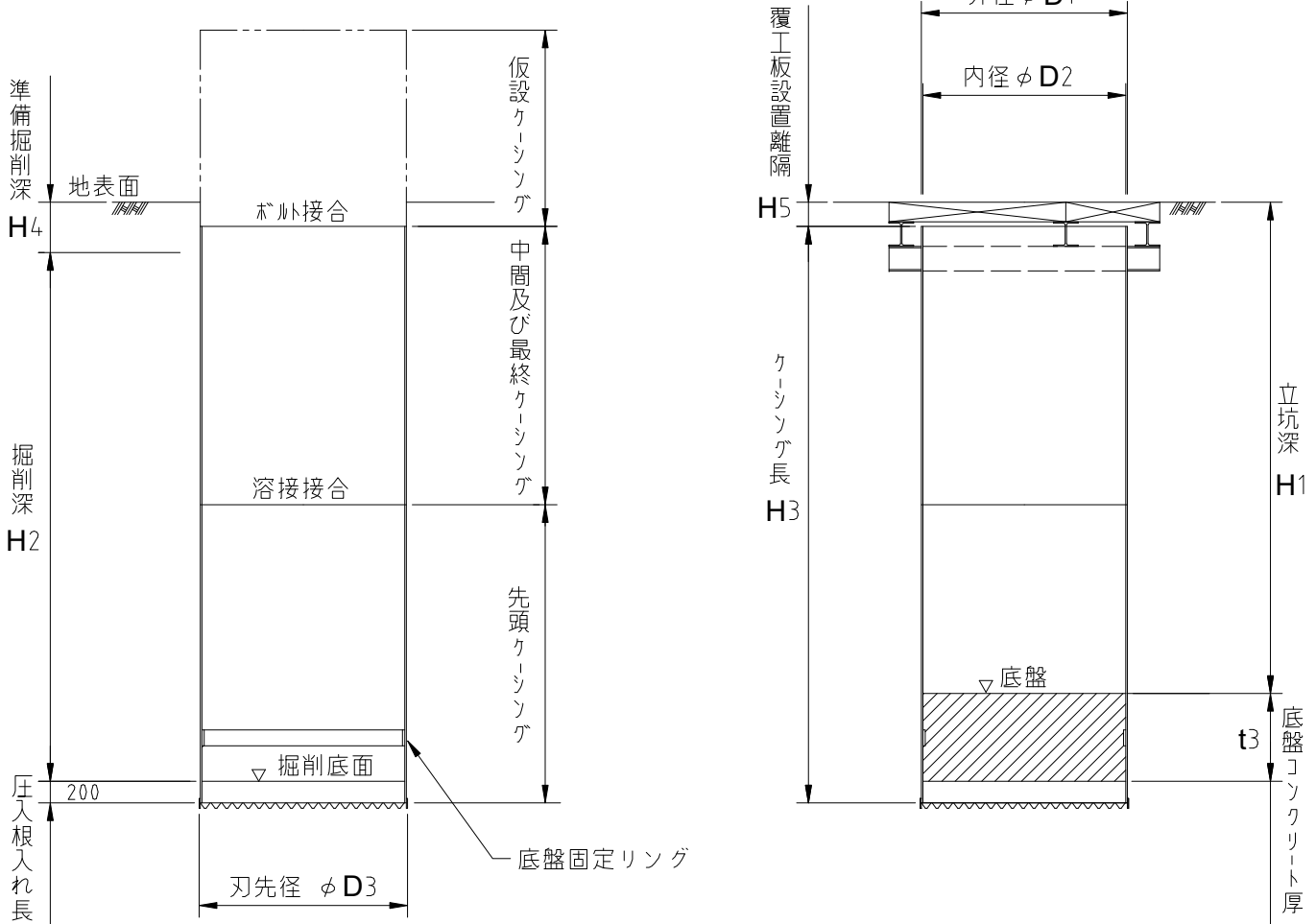
圧入掘削完了図
