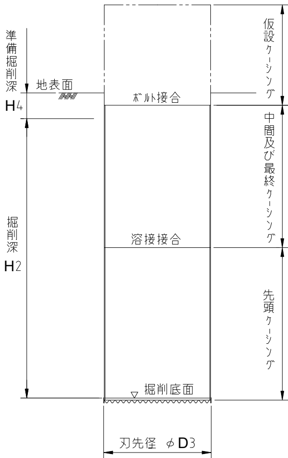
圧入掘削完了図
