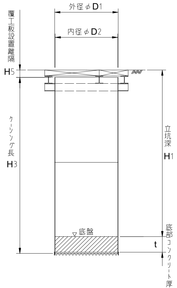
立坑構築完了図
